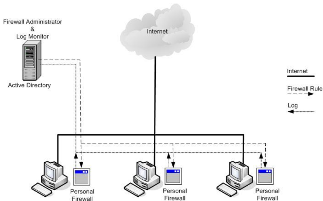
รูปที่ 7-1 โครงสร้างทางเครือข่ายของระบบที่ใช้ในการทดสอบ
