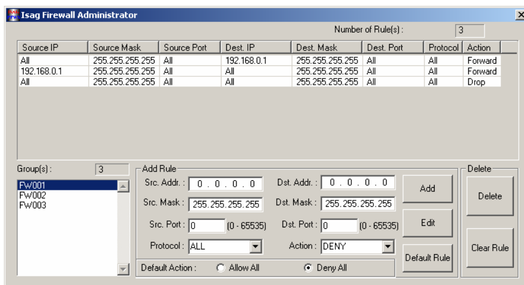
รูปที่ 7-2 โปรแกรมไฟร์วอลล์แอดมินิสเทรเตอร์
