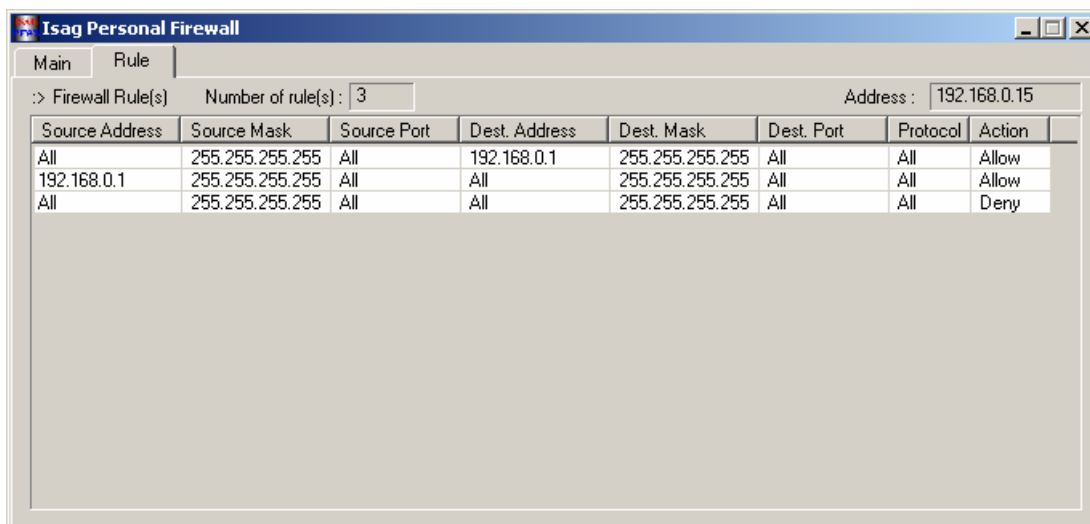
รูปที่ 7-4 แสดงกฎการฟิเตอร์ที่รับมาจากเซิร์ฟเวอร์
